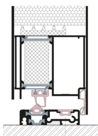
Próg aluminiowy
