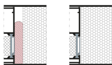
Osadzenie wypełnień
